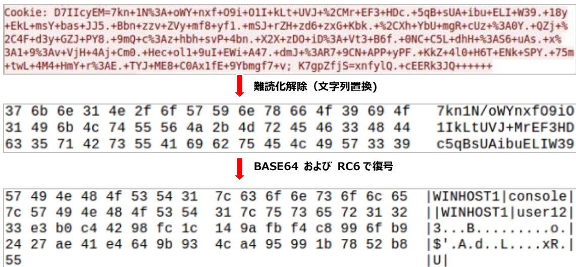
図 3-7 データ復号の流れ (Cookie ヘッダ)
