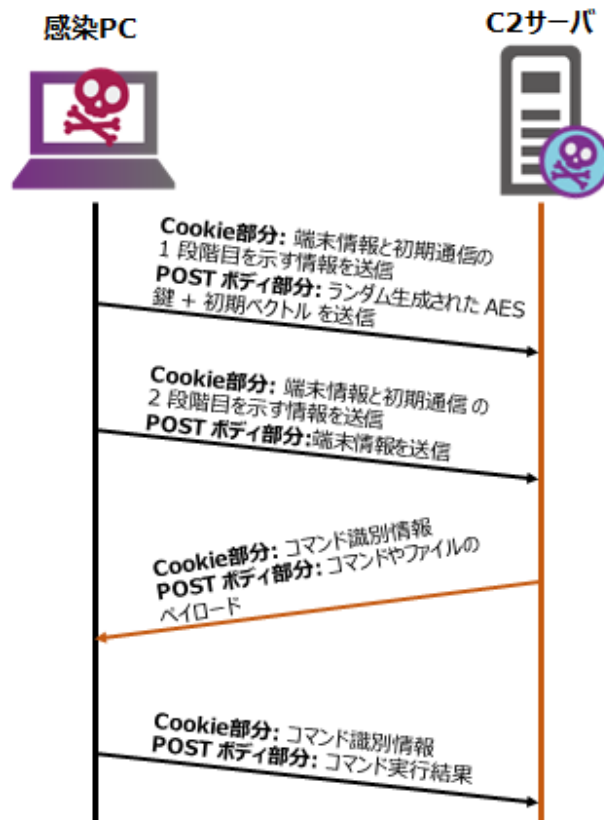
図 3-5 「WellMess」と C2 サーバとのやり取りの流れ
